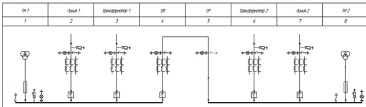
Проект №1. ЗРУ из 8 ячеек КРУ «Нексус» в здании размером 5700x11800 мм
