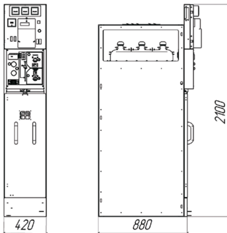
Камера КСО-300 на базе SL-12
