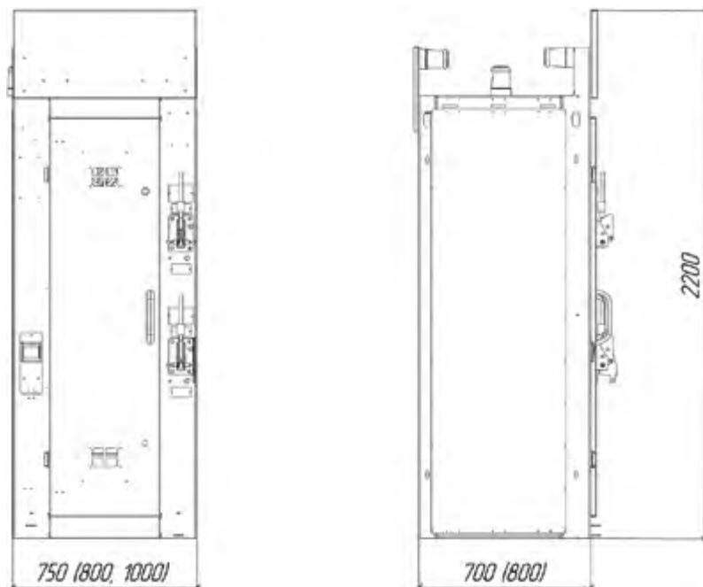
Камера КСО-300 на базе ВНА
