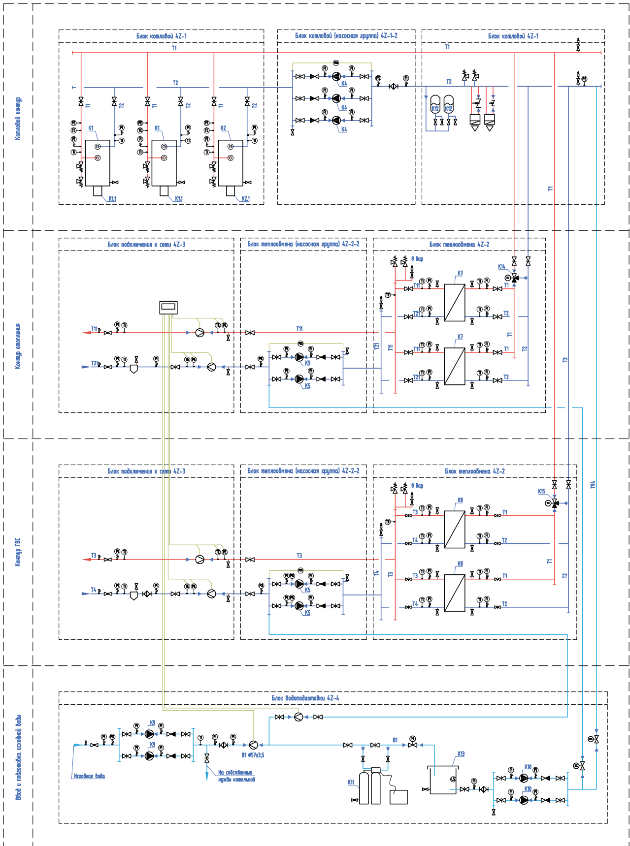
Схема тепломеханическая принципиальная
